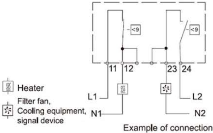
Thermostat ZR 011(NC/NO)
